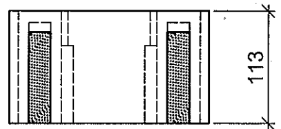
Schnitt B-B 1:5
