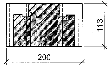
Schnitt A-A 1:5
