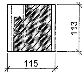
Schnitt A-A 1:5
