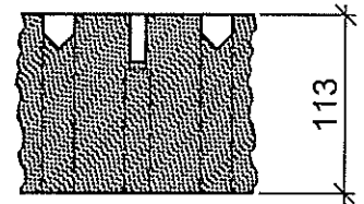
Schnitt C-C 1:5
