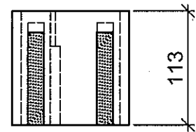
Schnitt B-B 1:5
