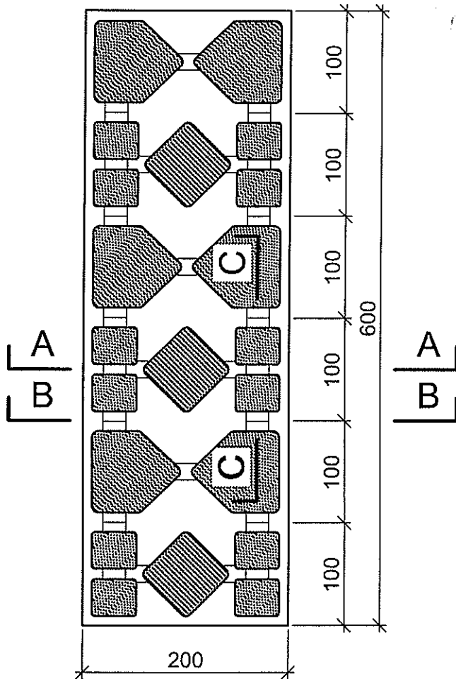
Draufsicht 1:5
