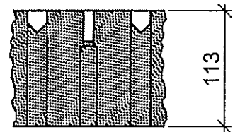
Schnitt C-C 1:5
