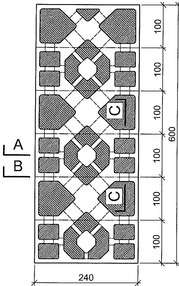
Draufsicht 1:5
