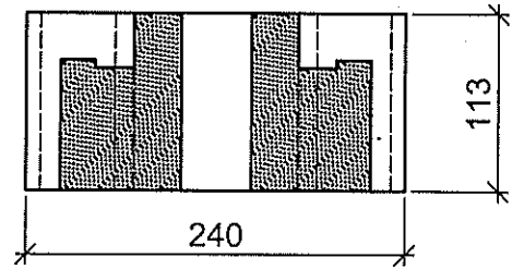
Schnitt A-A 1:5
