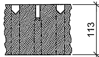
Schnitt C-C 1:5
